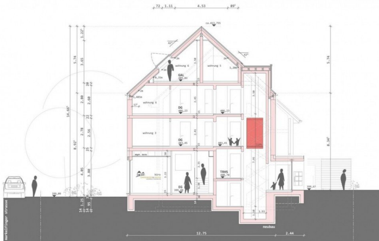
C-C Schnitt
