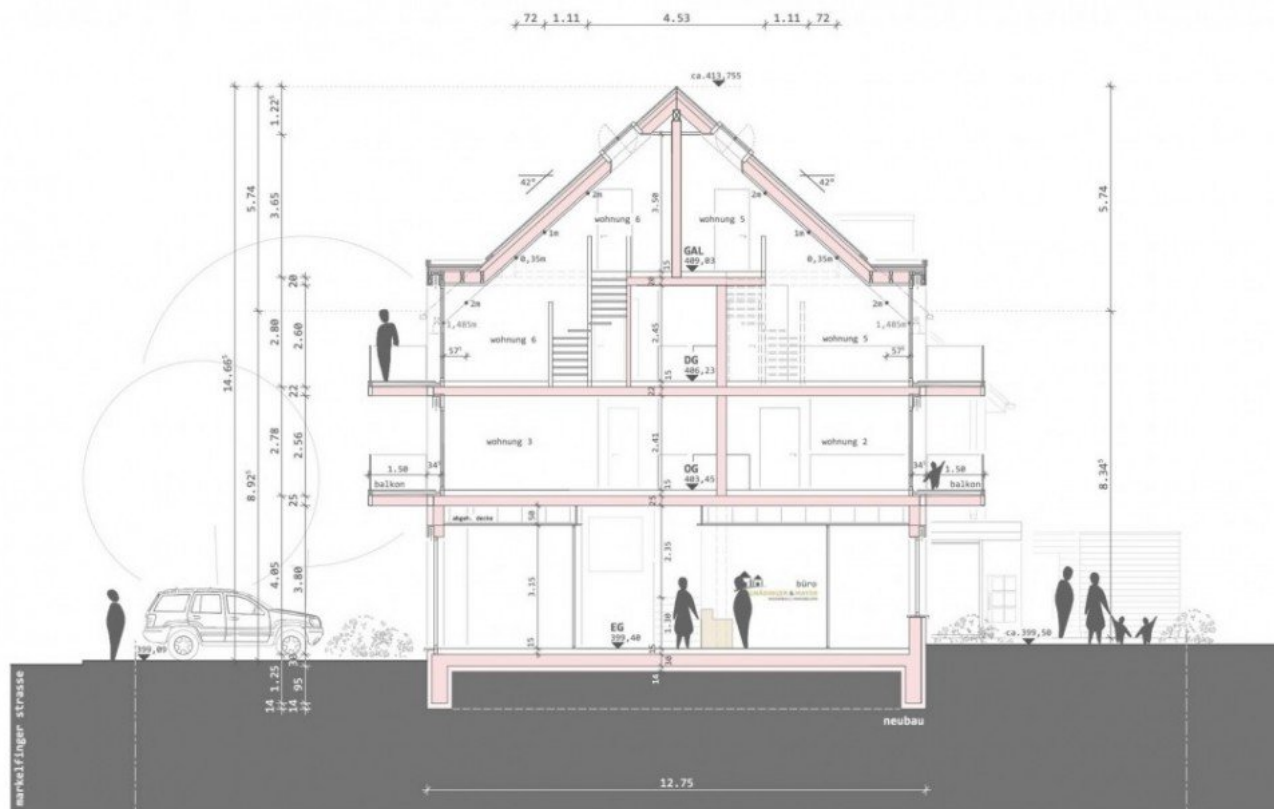
D-D Schnitt
