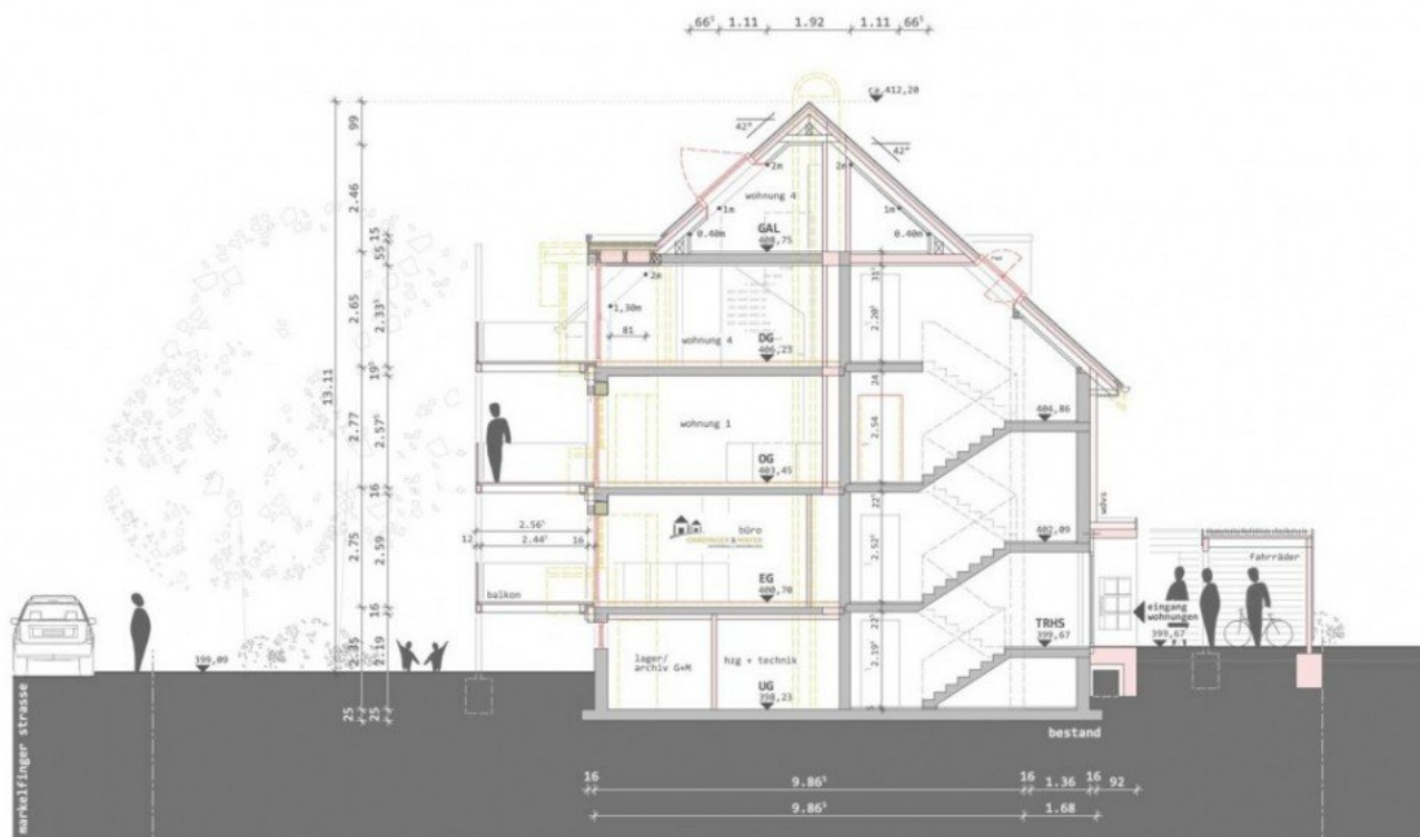
B-B Schnitt
