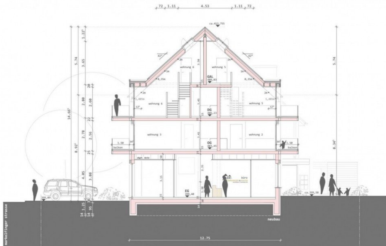
D-D Schnitt
