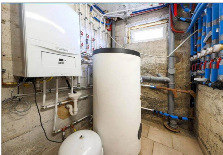
Zentralheizung
